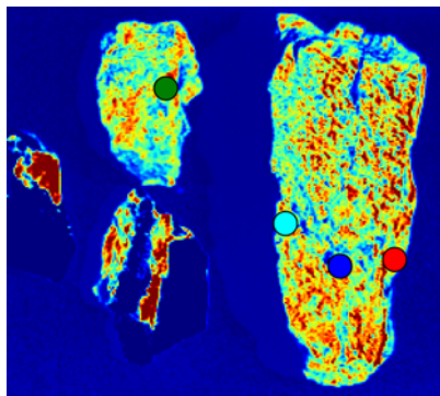
OLI
