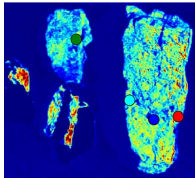
ETM+
